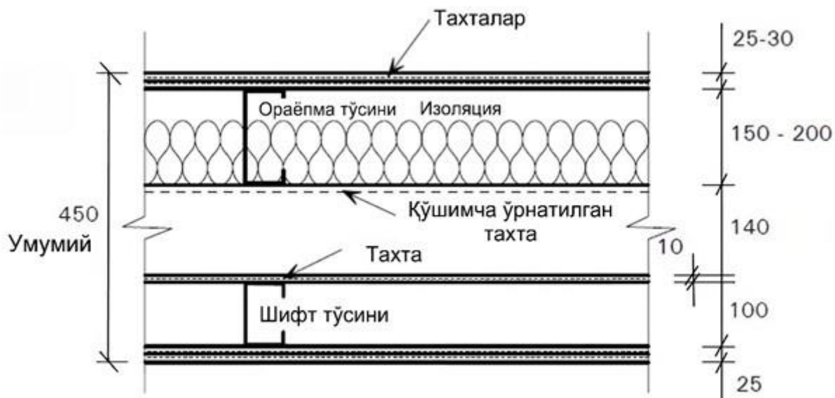
53-расм. Модулли меҳмонхона биноларидаги пол ва шифтнинг умумий қалинлиги
