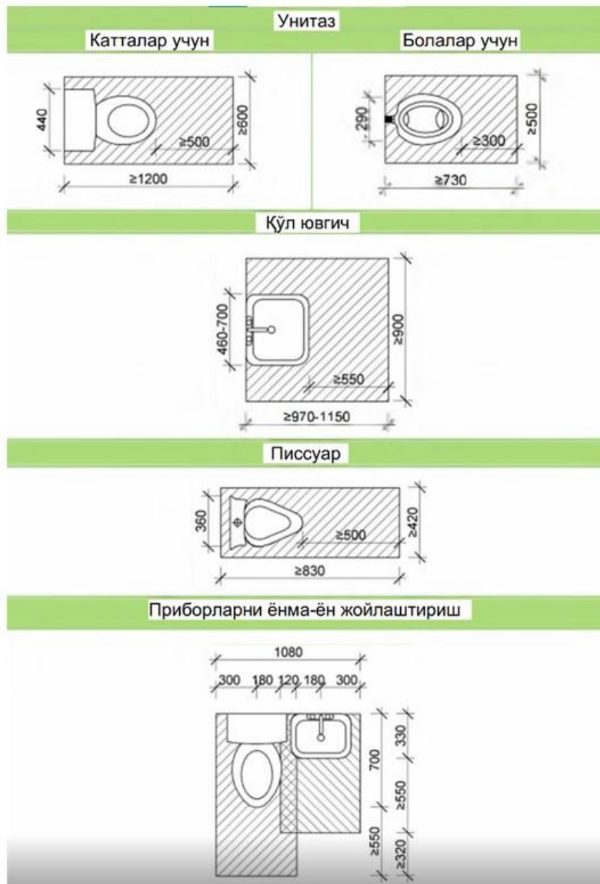
61-расм. Жамоат биноларидаги санитария узелларининг лойиҳавий (режавий) ечимларида қабул қилинган санитария-техник приборларнинг функционал зоналари (mm)
