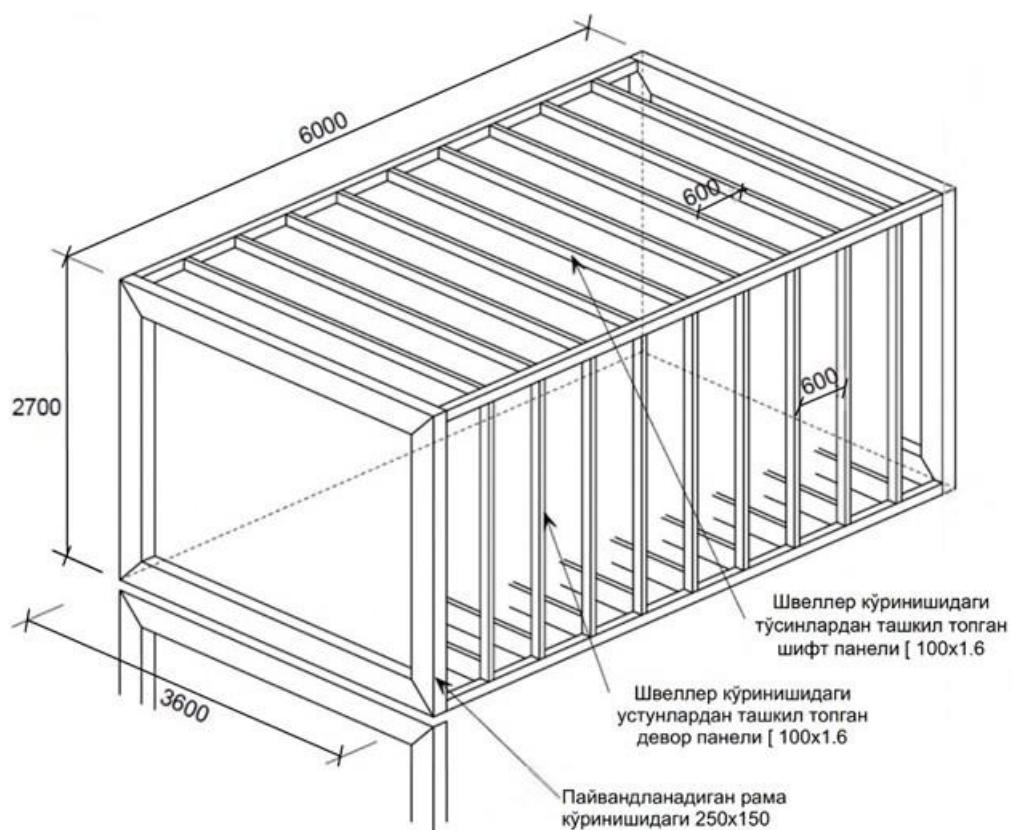
57-расм. Тўрт томонли модулнинг ўлчамлари
