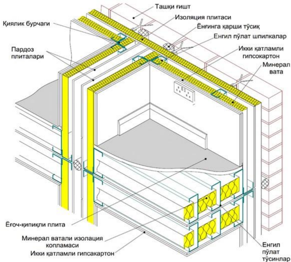
54-расм. Модулли меҳмонхона девори ва полининг элементлари
