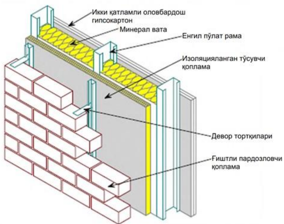
55-расм. Енгил пўлат деворларга маҳкамланадиган ғиштли пардозловчи қоплама ва девор элементлари
