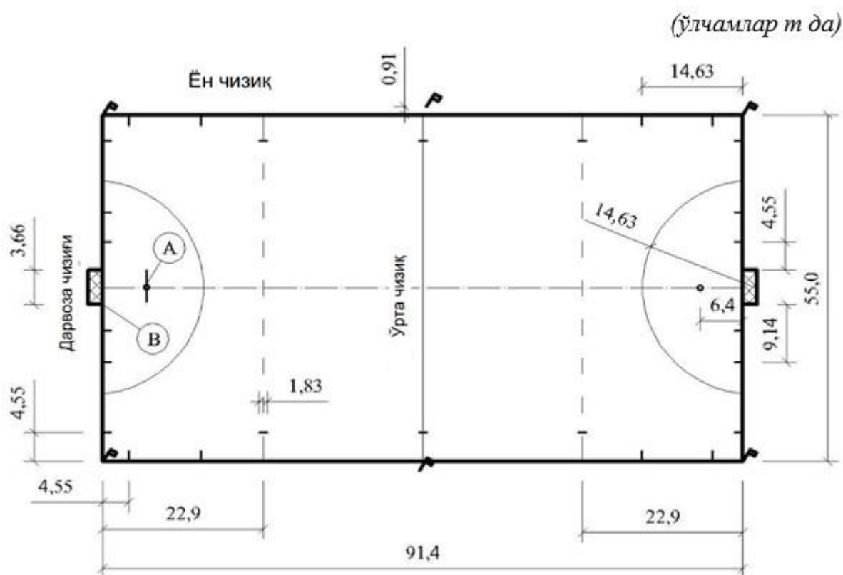
14-расм. Чим устида хоккей учун майдонча
