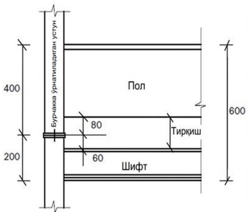
58-расм. Очик турдаги модуль шифти ва полининг умумий қалинлиги
