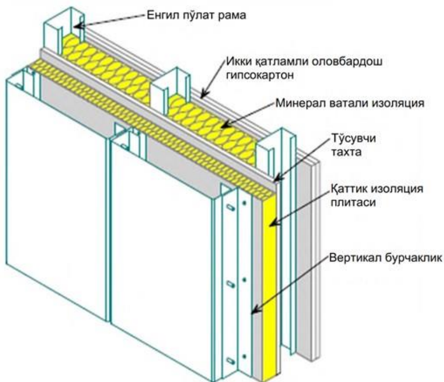
56-расм. Енгил пўлат деворларга маҳкамланадиган металл кассета
