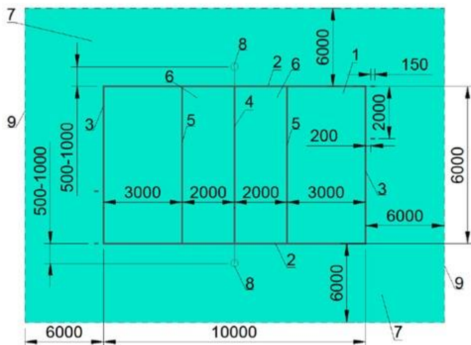
34-рasm. Ўтириб ўйналандиган волейбол учун спорт зонаси ва унинг чизиқлар билан белгиланиши
