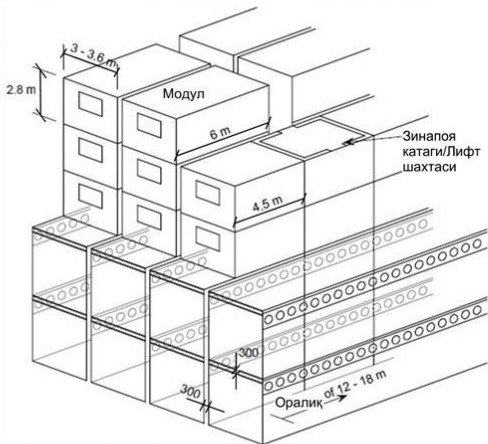
59-расм. Бирламчи структурали рамага таянувчи модулларнинг ўлчамлари ва улар конструкцияларининг оралиқ масофаси
