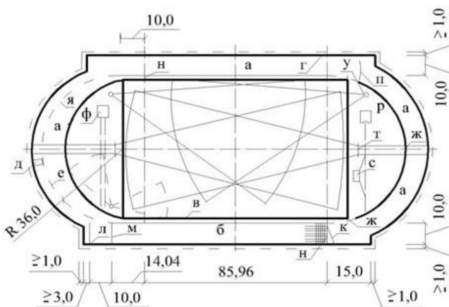
2-расм. Футбол майдони ва енгил атлетика йўлагига эга бўлган (битта марказли бурилишлар ва тўғри чизик бўйлаб 400 m узунлик бўйича югуриш учун) спорт ядроси (аренаси)нинг икки секторли режаси.
